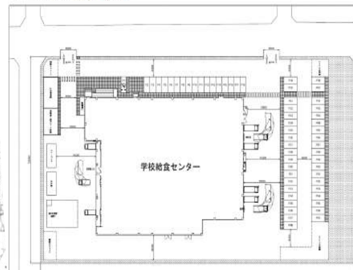
モデルプラン (施設配置図)
